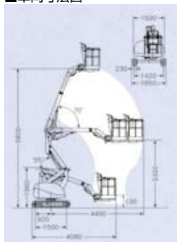
■車両寸法図
