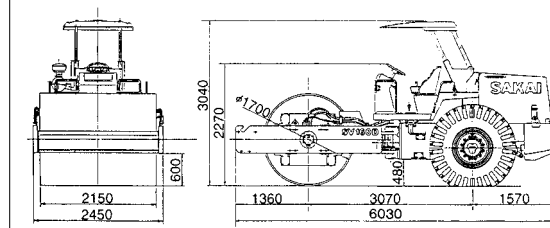
SV160D・SV160DV
