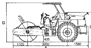
SV160D・SV160DV
