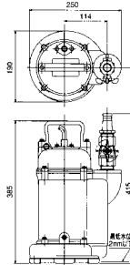
【UB-40】 外径寸法図
