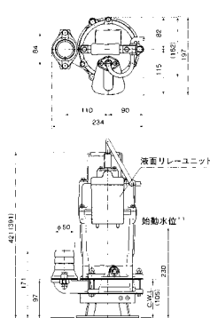
外径寸法図 (単位: mm)
