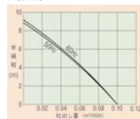
性能曲線
