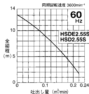
性能曲線
