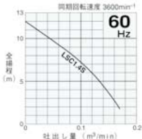
性能曲線
